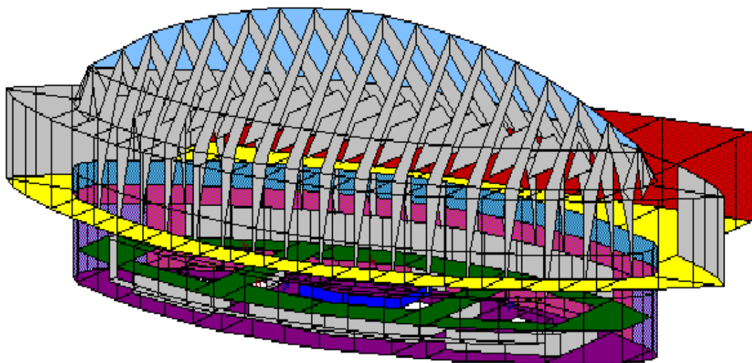
3D-Computermodell für die Simulation der raumakustischen Vorgänge
