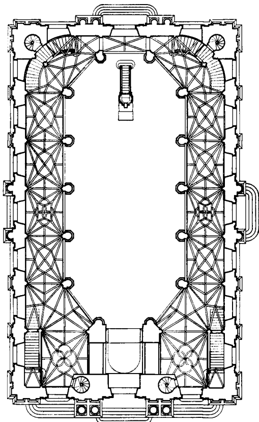
Grundriss
